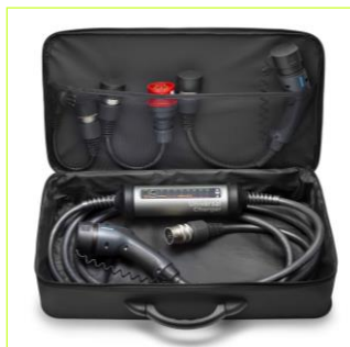
Súprava s nabíjacou jednotkou pre zapojenie do viacerých druhov elektrickej siete (230V/400V/WallBox) 98 357 837 80
